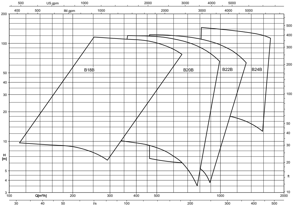
Raster_B Impeller @960rpm / 1
