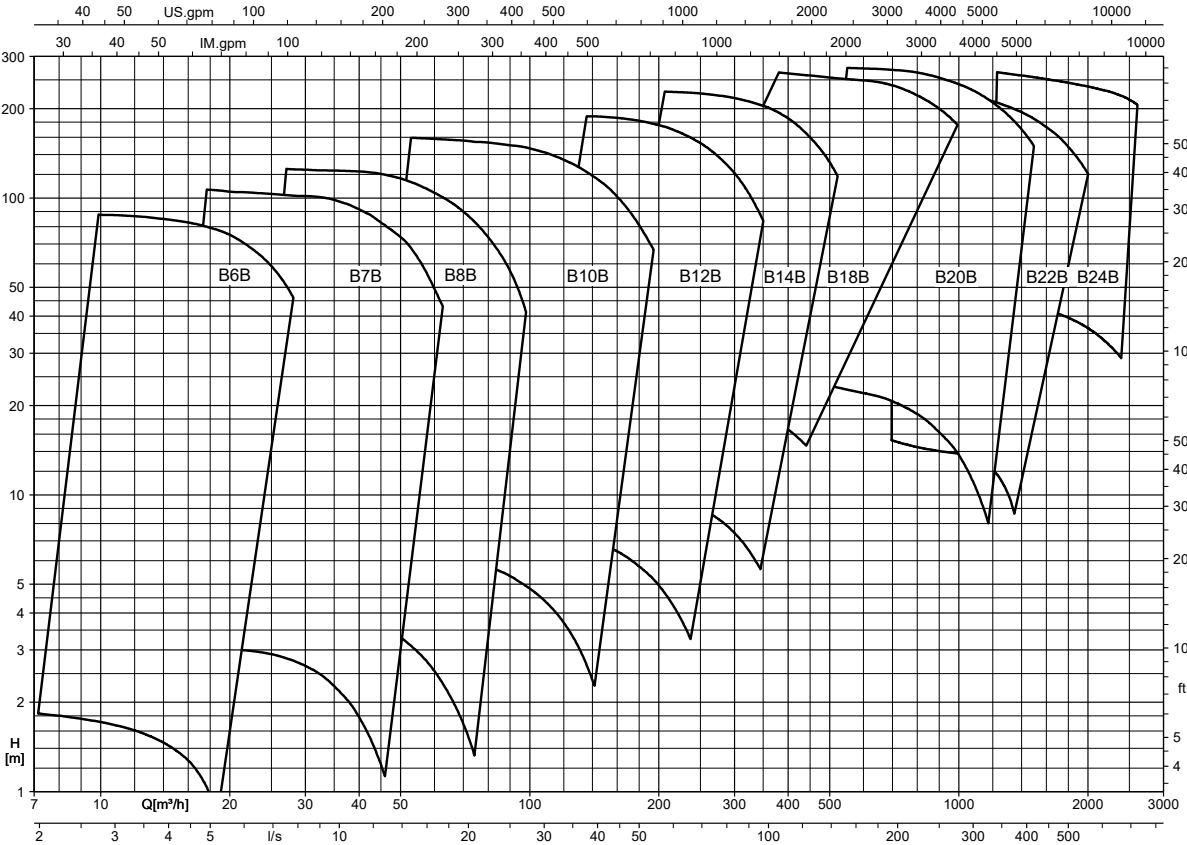
Raster_B Impeller @1450rpm / 1
