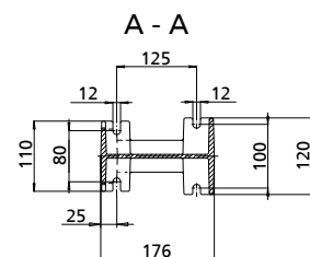
Pump flange DN 2 ISO 7005 PN 10/16 DIN 2501 PN 10/16
